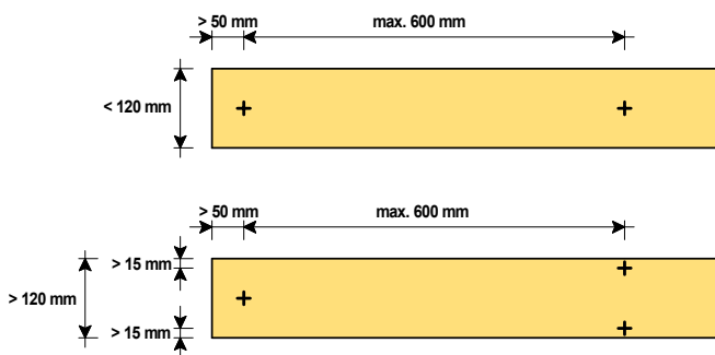
Tekening 8. Maatvoering bevestigingspunten.
