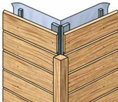
Tekening 5. Voorbeeld open gevelbekleding, afgeschuinde delen met mogelijke hoekoplossing.
