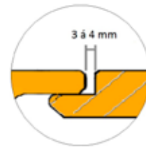
Tekening 9. Voldoende expansieruimte aanhouden tussen delen.
